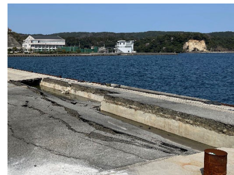
物揚場背後の沈下
