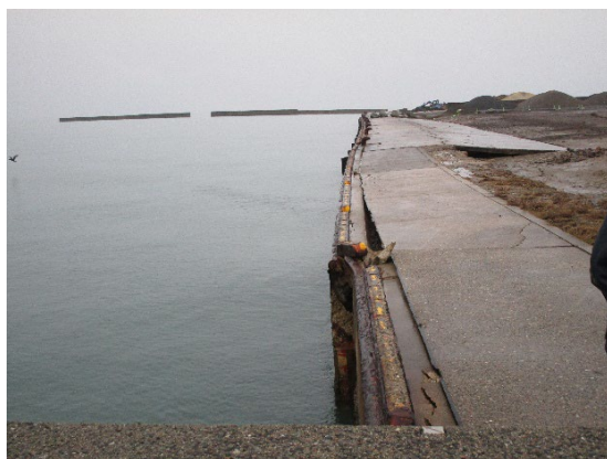
岸壁のズレ、岸壁背後の沈下
