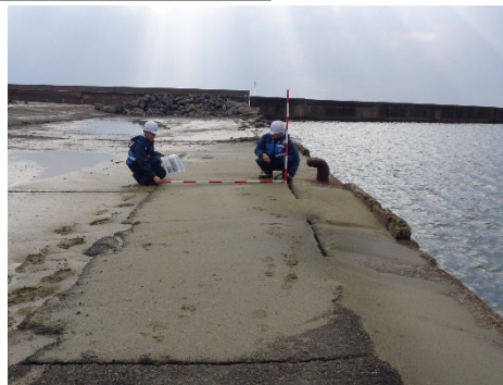
物揚場の傾斜・噴砂
