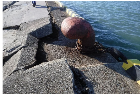
上部工の損傷
